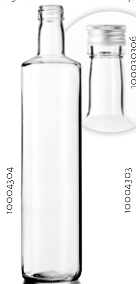
LÁHEV DORIKA 750 ml výška 308 mm
